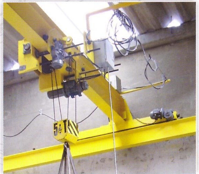
Puente Grúa Monoriel con Carro Testero - Emino Carros Testereros Jgo × 2 und - 5.000Kg
