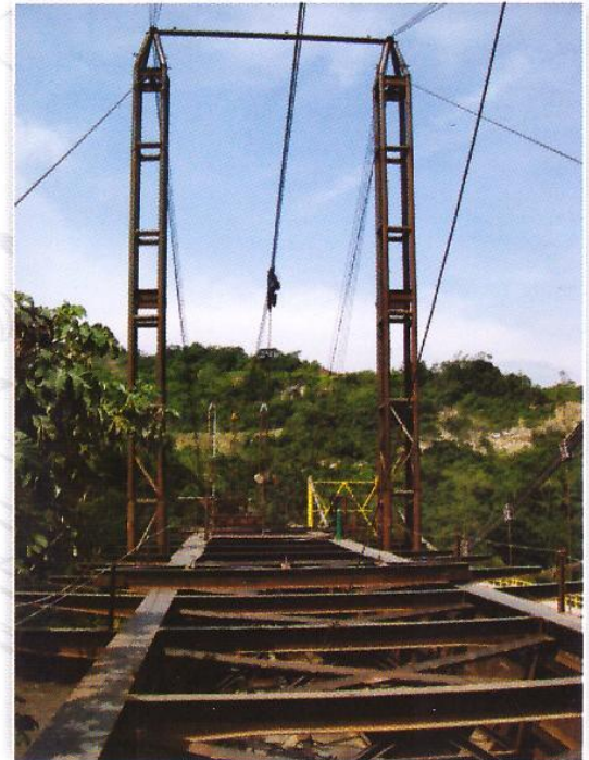
CONCREARMADOS - Obra Hidrosogamoso Teleféricos 10.000Kg
